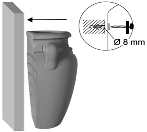
ANTIK Wand-Amphore Amphore antique murale Antique wall amphore Ánfora de pared ANTIK Anfora da parete anticata
